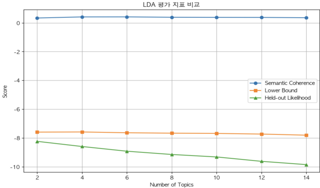
그림 1. Semantic Coherence, Lower Bound, Held-out Likelihood에 따른 최적 토픽 수
